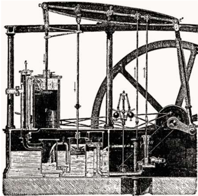
Figura 22. La máquina de vapor de Watt.
